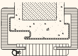
Reno-Zarge SOFT Verkleidungsbreite 80 mm
