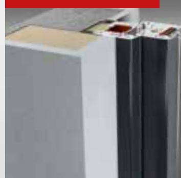
Konventionelles Fenster
